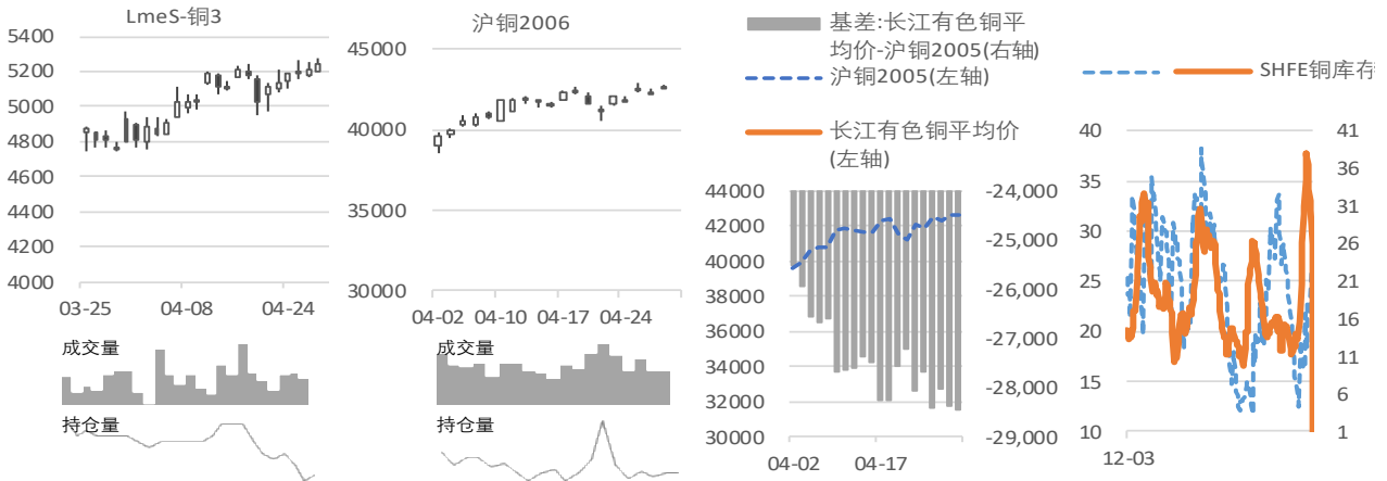
图 3：铜的价格、成交量、持仓量、基差和库存
