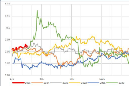
Au/Ag季节性
