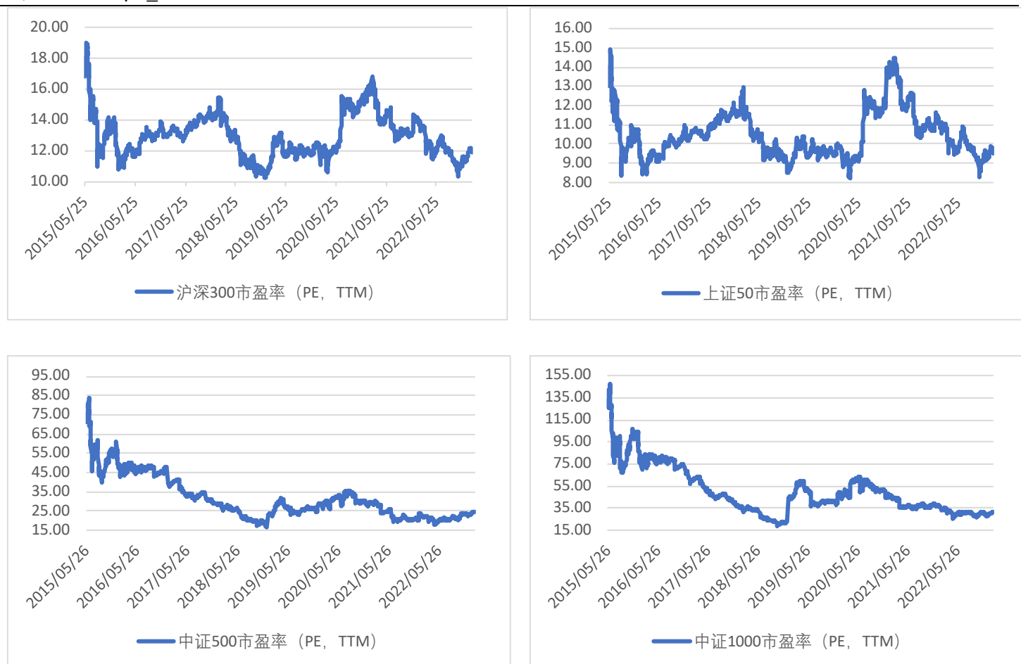
图 8 估值 (pe_ttm)
