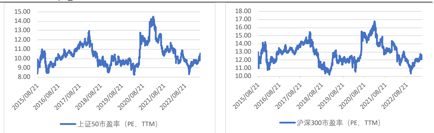
图 10 估值 (pe_ttm)
