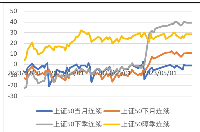
图9 股指基差
