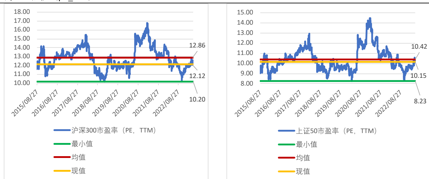
图 10 估值 (pe_ttm)
