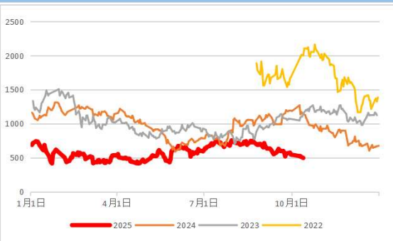
LU-FU季节性
