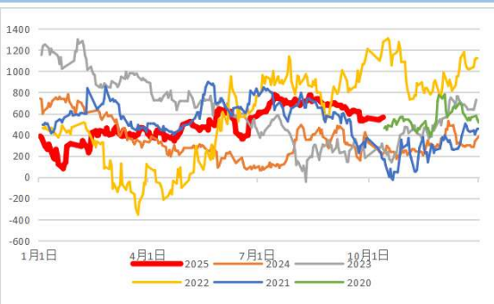
BU-FU季节性
